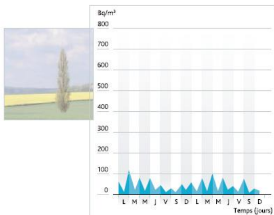
Figure 3. Exemples de variation quotidienne des concentrations d'un lieu à l'autre en fonction des caractéristiques géologiques
