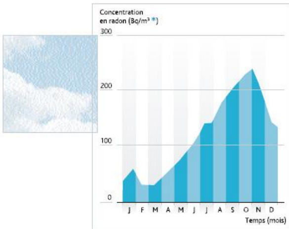
Figure 1. Exemple de variation mensuelle de la concentration en radon dans le Massif-Central
