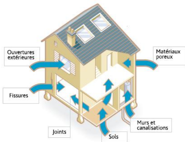
Figure 4. Voies d'entrée du radon dans une maison
