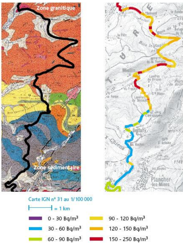
Figure 2. Exemple de variation des concentrations d'un lieu à l'autre en fonction des caractéristiques géologiques
